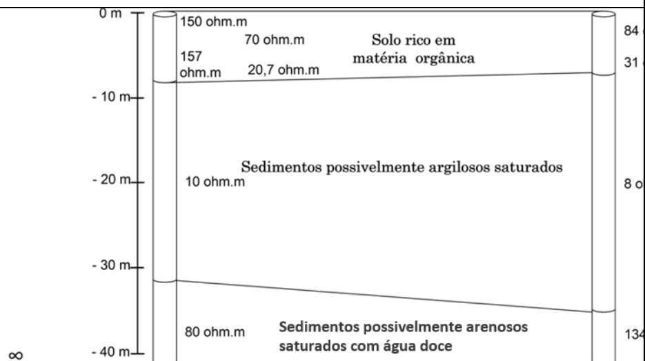
Figura 48 - Modelo geoeletrico interpretado inferindo as possíveis litologias e níveis de aquífero na área de Jardim Aguapeu em Itanhaém, SP.
