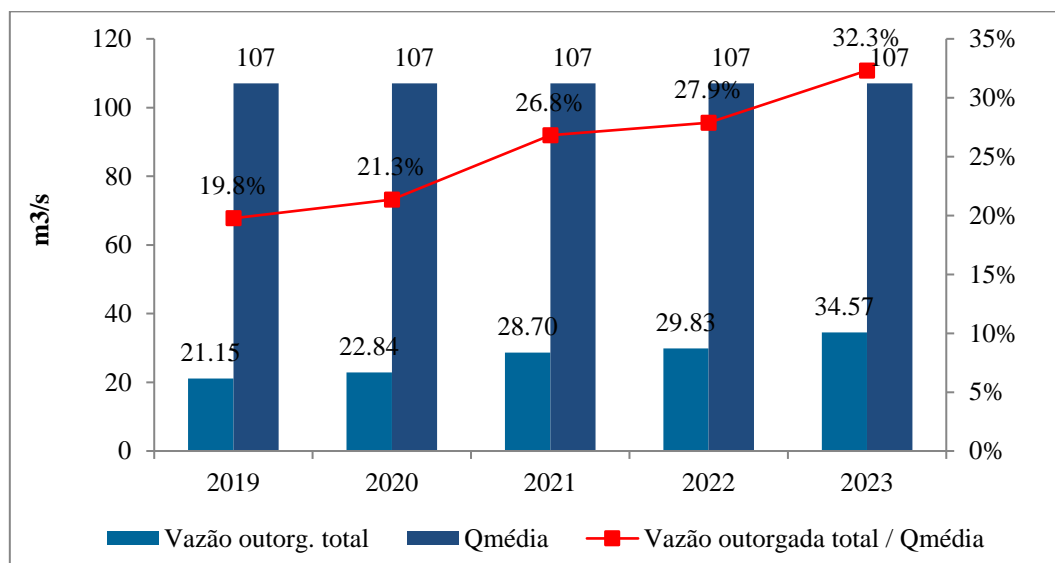
Figura 31 – E.07-B - Vazão outorgada total (superficial e subterrânea) em relação ao Q_{m\u00e9dio} : %. Fonte: DAEE, 2024.
