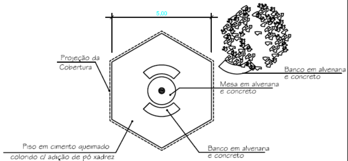
PLANTA ESC. : 1 : 100
