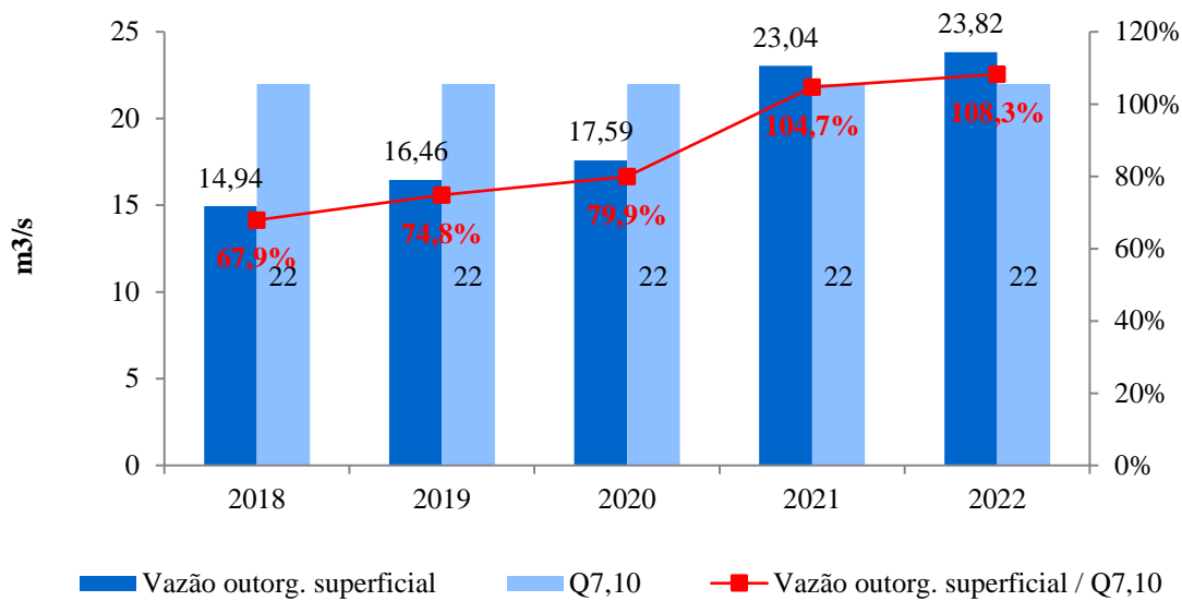
Figura 32 – E.07-C - Vazão outorgada superficial em relação a vazão mínima superficial (Q 7,10 ): %. Fonte: DAEE, 2023.
