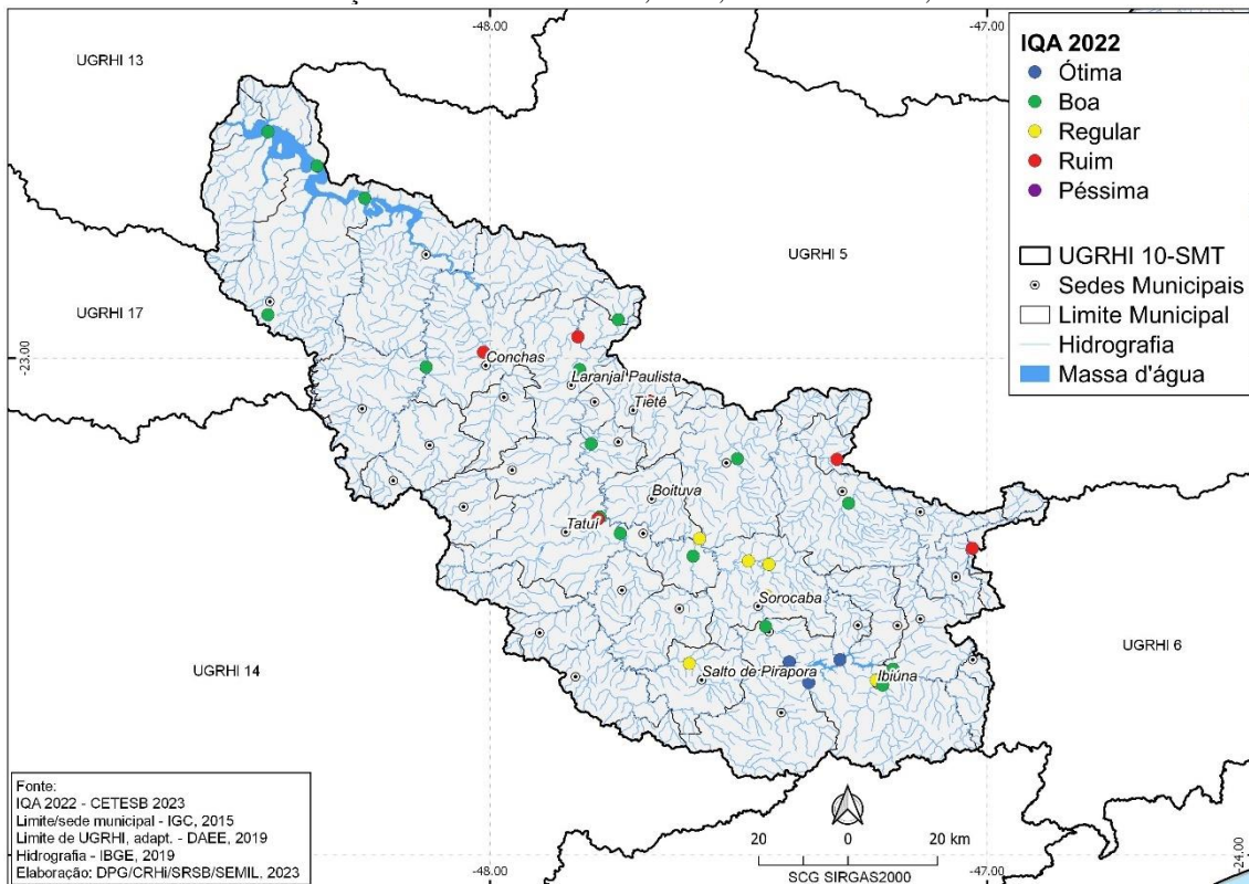
Figura 60 - Resultados do Índice de Qualidade da Água (IQA) na UGRHI 10 para o ano de 2022. Elaboração: DPG/CRHi/ SEMIL, 2023, Fonte: CETESB, 2023.
