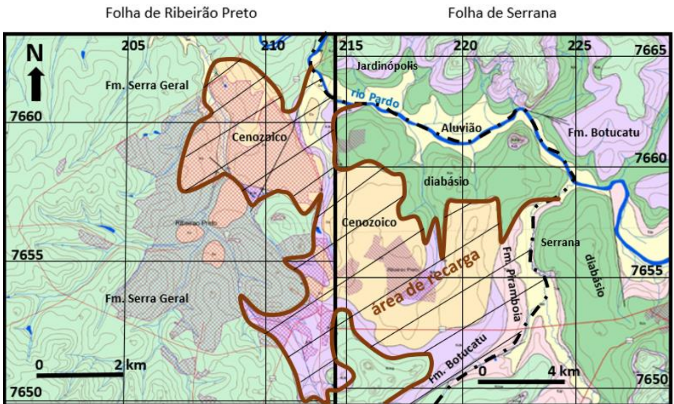
Figura 1 – Mapa geológico das folhas de Ribeirão Preto e Serrana. Adaptado de Sinelli et al. (1973). A área hachurada é a área de recarga do SAG.
